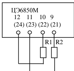
Рисунок 4.4- Схема подключения резисторов растяжки
